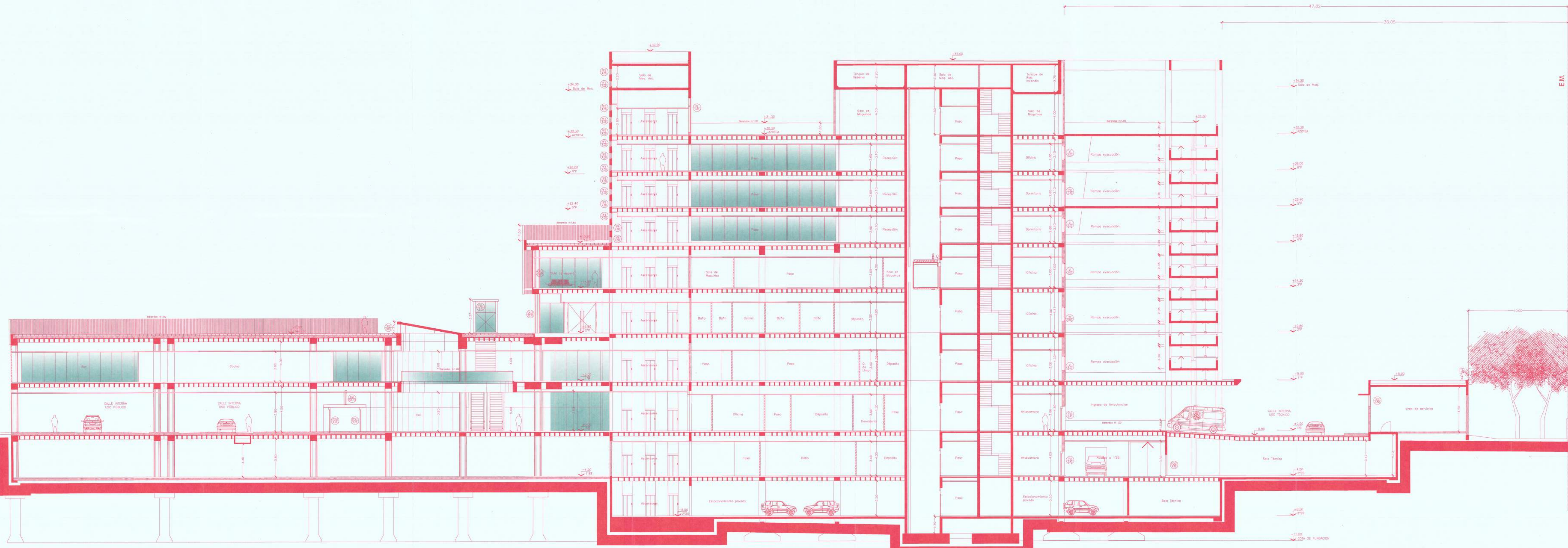
CORTE BB
