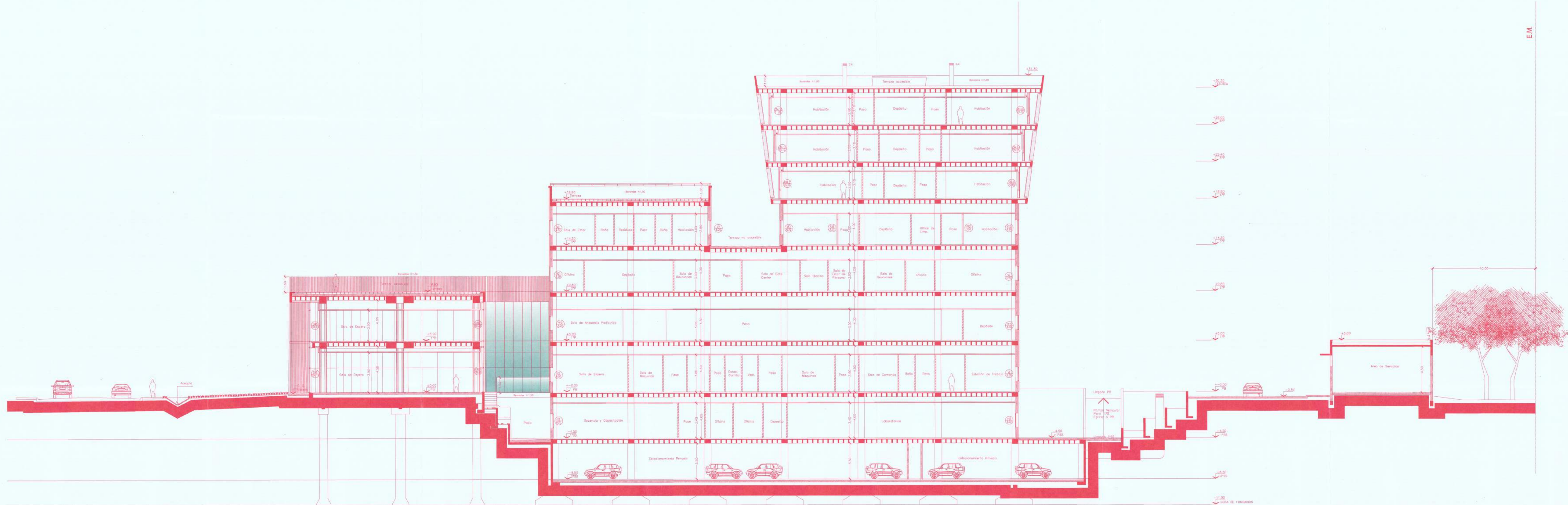
CORTE AA
