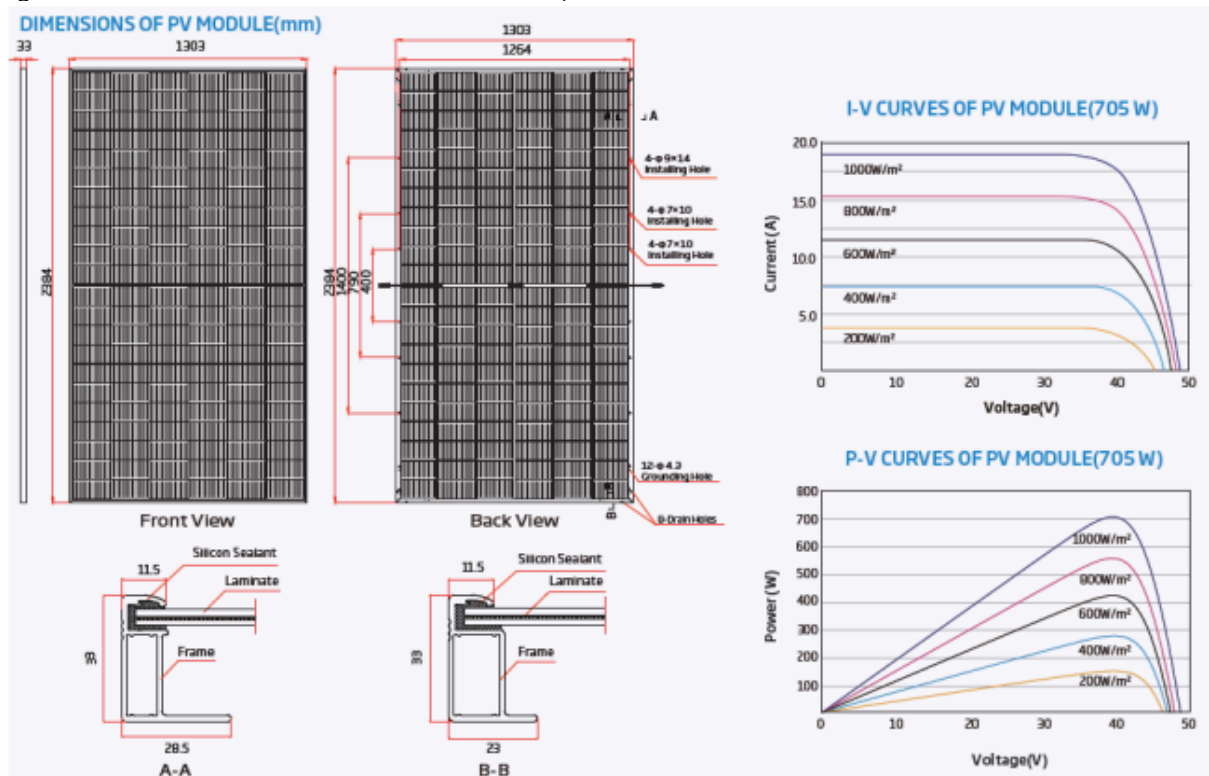
Imagen 3: Detalles de las dimensiones del módulo y curvas características
