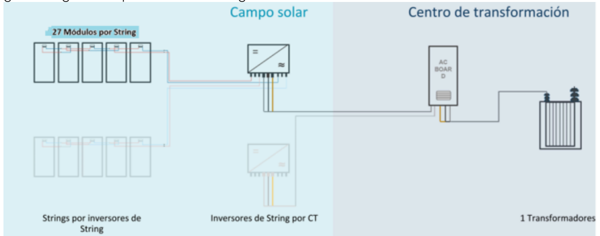
Imagen 2: diagrama simplificado de la configuración eléctrica
